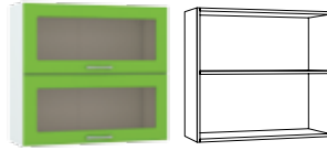
Шкаф навесной 800 гориз. 2 витрины (кроме кухонь Адель, Жанна) 800 x 318, В 680 мм
