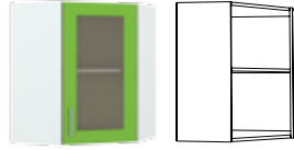
Шкаф навесной угловой витрина (кроме кухонь Адель, Жанна) 598 x 598, В 680 мм
