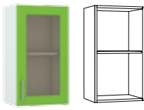
Шкаф навесной 400 витрина 400 x 318, В 680 мм
