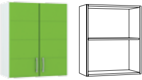
Шкаф навесной 600 2 двери (возможность установки сушики) 600 x 318, В 680 мм
