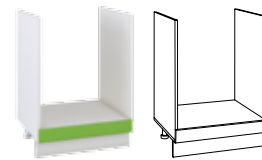
Стол 600 для духовки и вар. панели 600 x 600, В 836 мм
